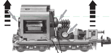
6518 ERSATZSCHLEIFKOHLEN SPARE BRUSHES BALAIS DE RECHANGE
